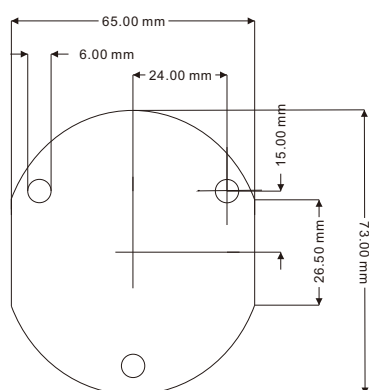
底座
