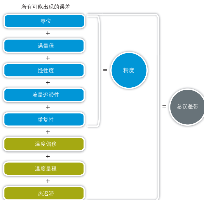
图 1: 总误差带与精度
