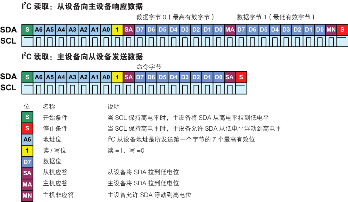
图 7：传感器 I 2 C 读和写命令
